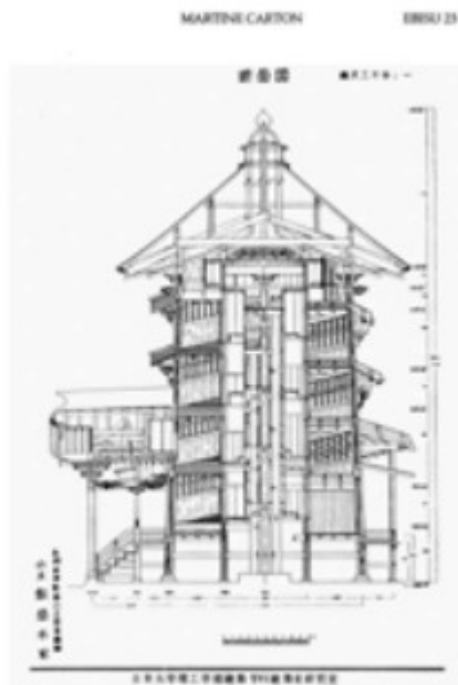
Illustration 4 : Structure du Sazae-dô d'Aino wakamatsu, coupe, Kōyasan, Buigi, Laboratoire d'histoire de l'architecture, Université Nihon.
